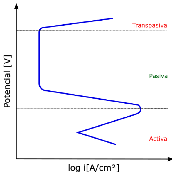
Figura 1. Diagrama de polarización en función del voltaje y la densidad de corriente.
