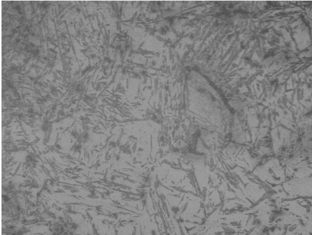
Figura 3. Micrografía de martensita de un acero 1045 templado en agua, 400 x ataque químico con nital al 2%.
