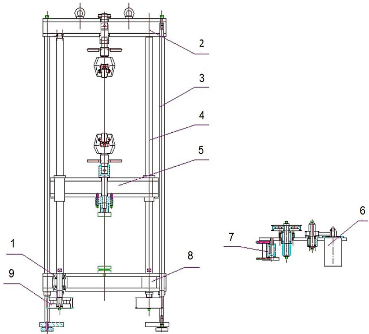
1. Rodamiento 2. Mecanismo de transmisión 3. Motor 4. Mecanismo tensor 5. Mesa de trabajo 6. Cabezal móvil 7. Tornillo de bolas 8. Columna 9. Cabezal superior
