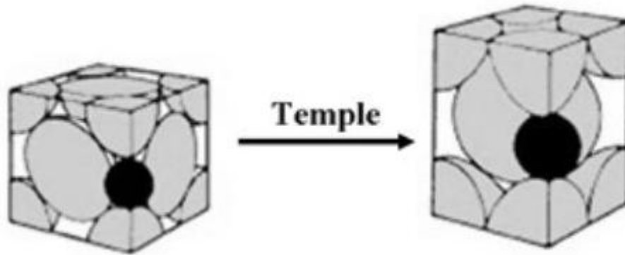
Figura 4. Celda cúbica de la austenita y celda tetragonal centrada en el cuerpo de la martensita.
