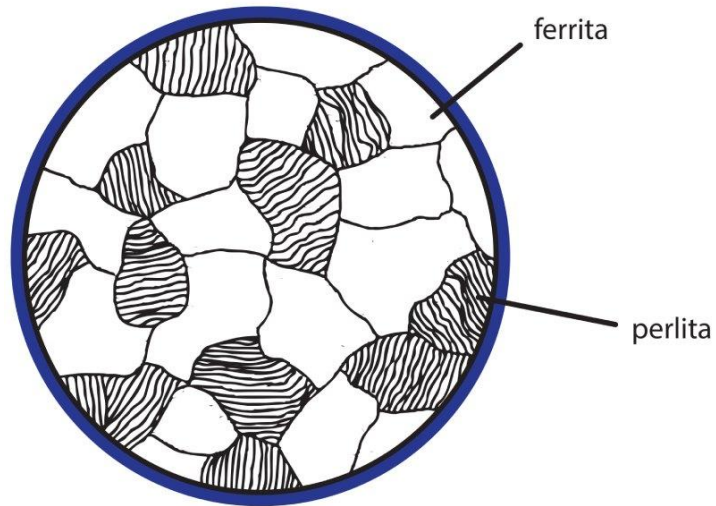
Figura 2. Esquematzación de la microestructura del acero al carbono.
