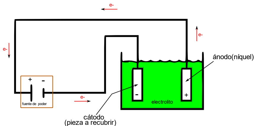
Figura 1. Diagrama de conexión de la celda de electrodeposición.
