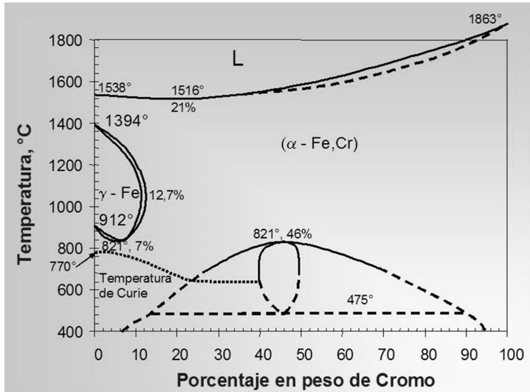
Figura 17. Diagrama de fases Fe-Cr
