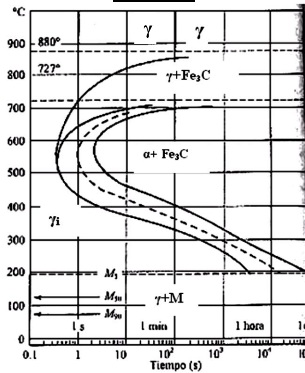
Figura 10.- Acero con 1.13% de C
