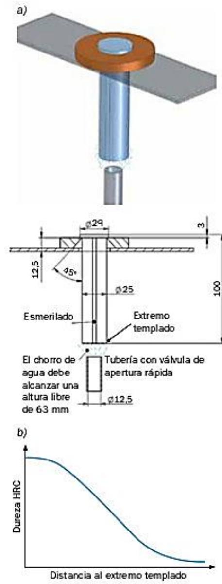
Figura 9. Ensayo de templabilidad Jominy
