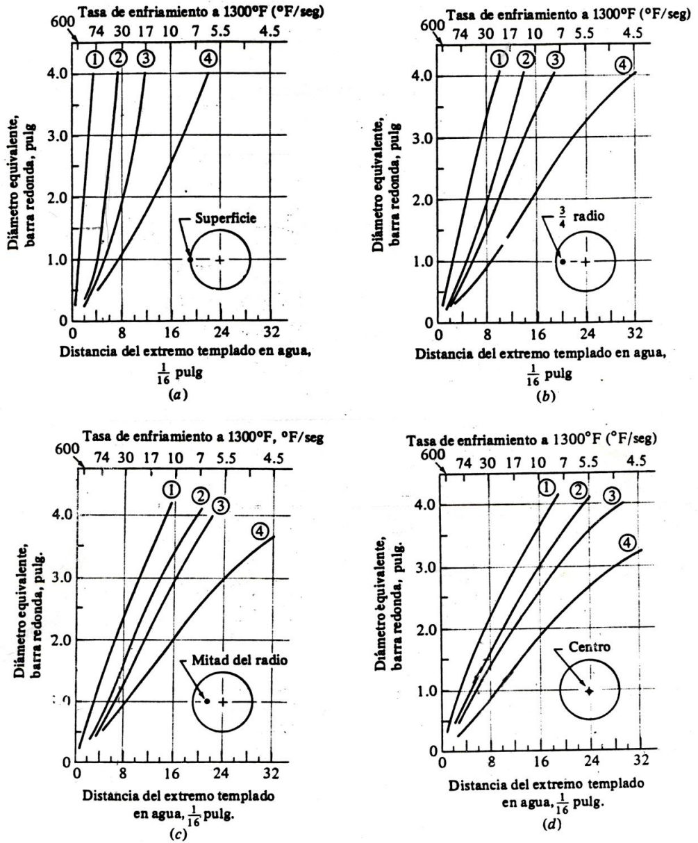
Figura 15.- Relaciones entre las tasas de enfriamiento en barras redondas y en localizaciones Jominy
