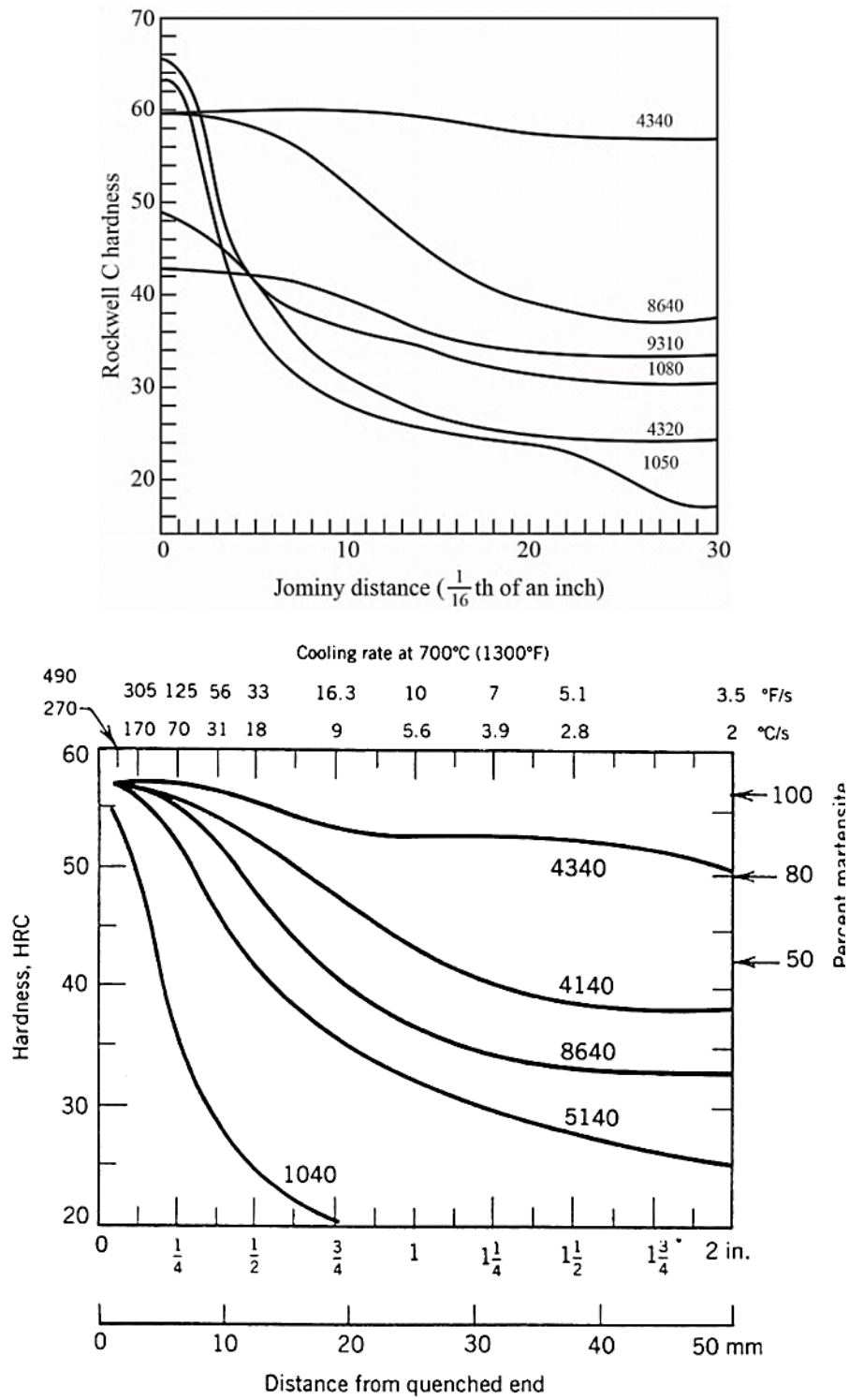
Figura 16.- Curvas de templabilidad para distintos aceros
