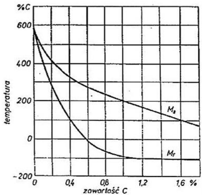
Figura 13. Temperaturas M_s y M_f en función del contenido de carbono
