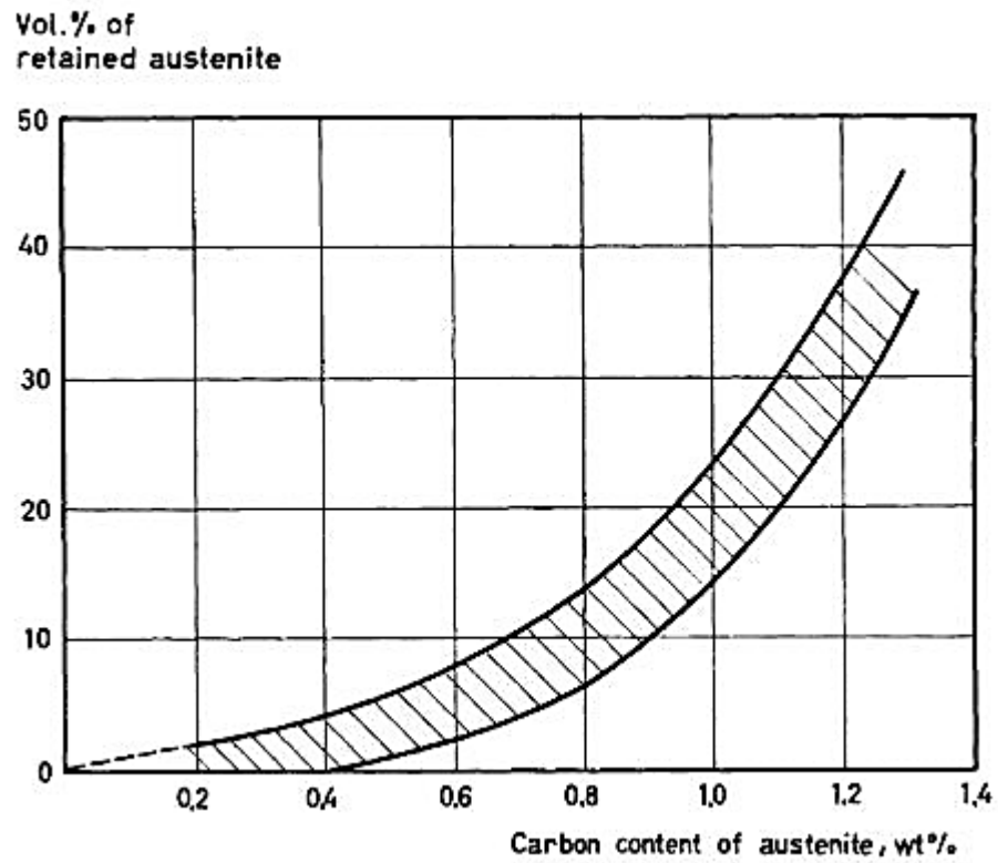
Figura 14. Variación de la cantidad de la austenita retenida en función del contenido de carbono
