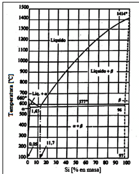
Figura 6.- Diagrama de fases aluminio-silicio
