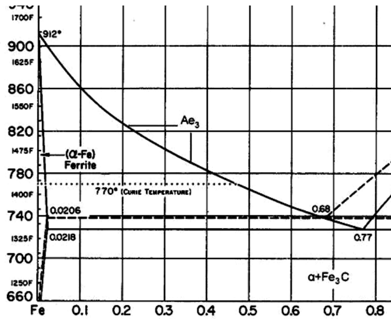
Figura 2. Zona hipoeutectoide
