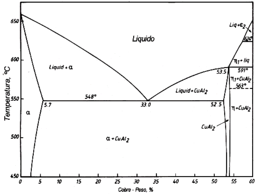
Figura 5.- Diagrama de fases aluminio-cobre
