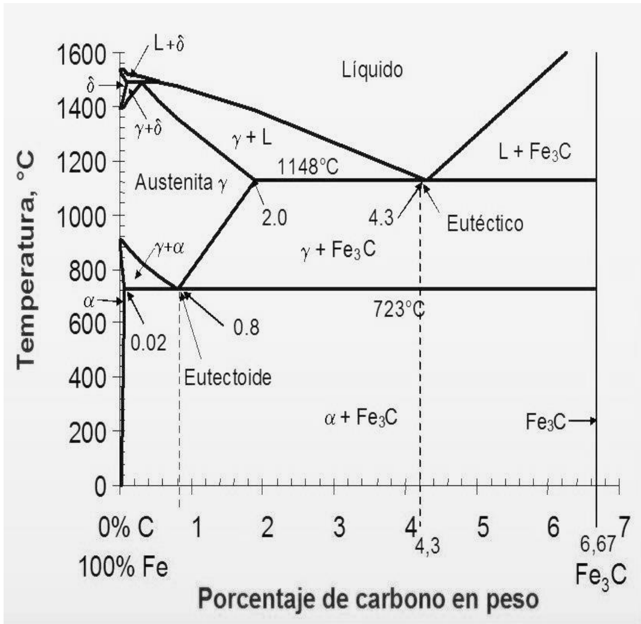
Figura 1.- Diagrama de fases Fe- Fe 3 C
