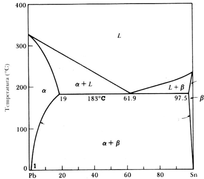
Figura 7.- Diagrama de fases Pb-Sn
