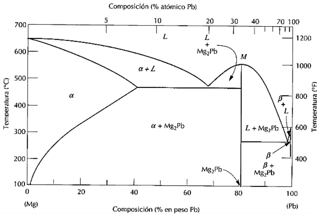
Figura 8.- Diagrama de fases magnesio-plomo
